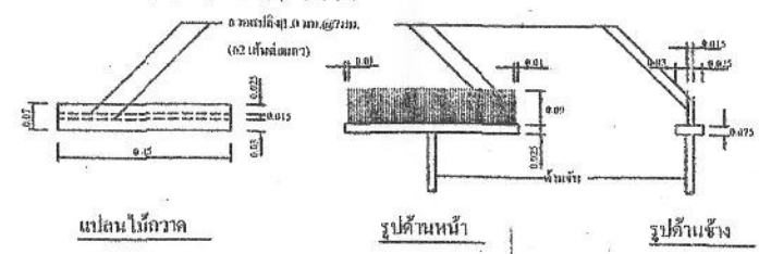
แบบขยายไม้ทาบคานผิวพื้น คสส.
